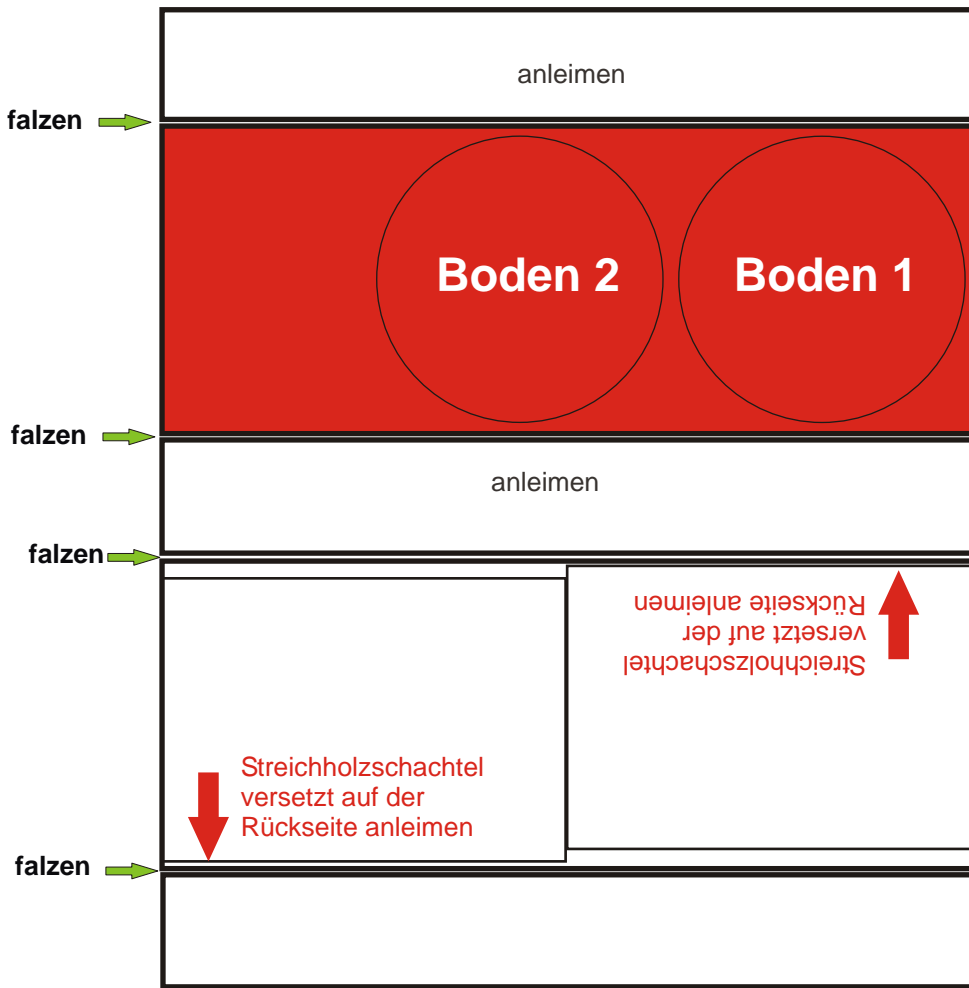
Die Streichholzschachteln sind etwas schmaler als die entstehende Bodenschachtel. Sie werden etwas versetzt in der Schachtel angeleimt.
